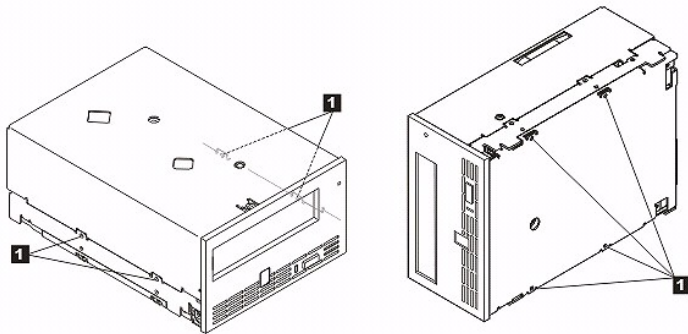
Abbildung 4. Befestigungslöcher am Bandlaufwerk
