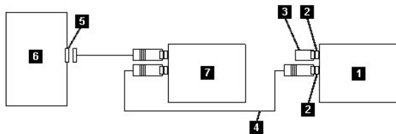
Abbildung 9. Mehrere SCSI-Einheiten anschließen
