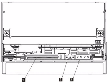
Abbildung 1. Rückansicht des Bandlaufwerks
