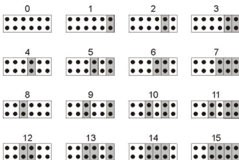
Abbildung 2. Kontaktstifte des SCSI-Anchlusses
