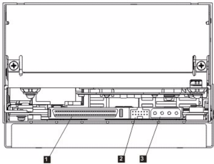
Abbildung 4. Rückwand des internen Bandlaufwerks
