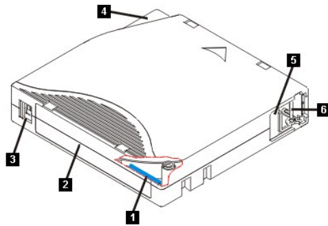
Abbildung 3. LTO Ultrium 400-GB-Datenkassette
