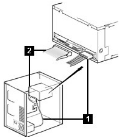
Abbildung 5. Netzkabel und SCSI -Kabel anschließen
