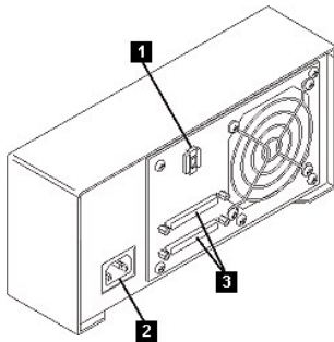
Abbildung 5. Rückwand des externen Bandlaufwerks
